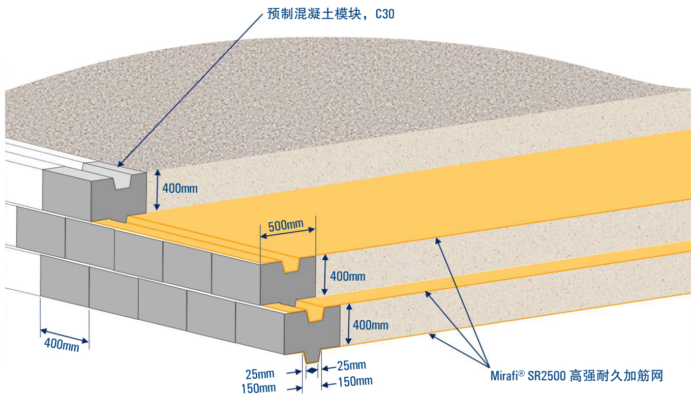
> 图2. 包含面板、筋材和结构填土的加筋土挡墙示意图。
